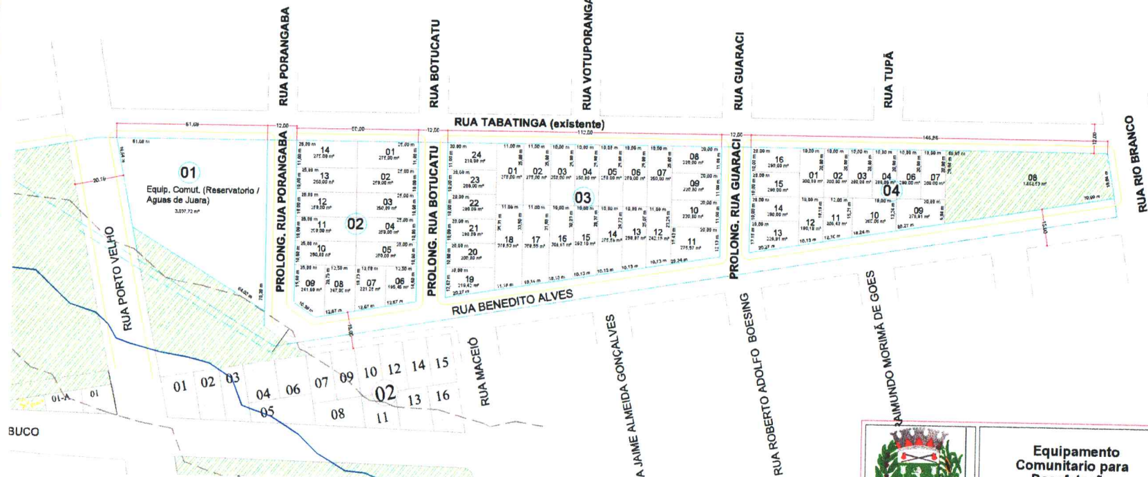
PLANTA - PROPOSTA DE DESAFETAÇÃO DE ÁREA DE EQUIPAMENTO COMUNITÁRIO Escala - 1/750
